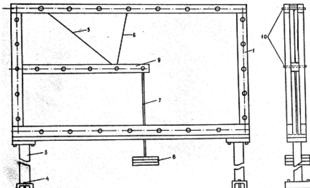
Сүрет 1. Стержендік жүйелерді созылу – сығылу сынау үшін қондырғы
