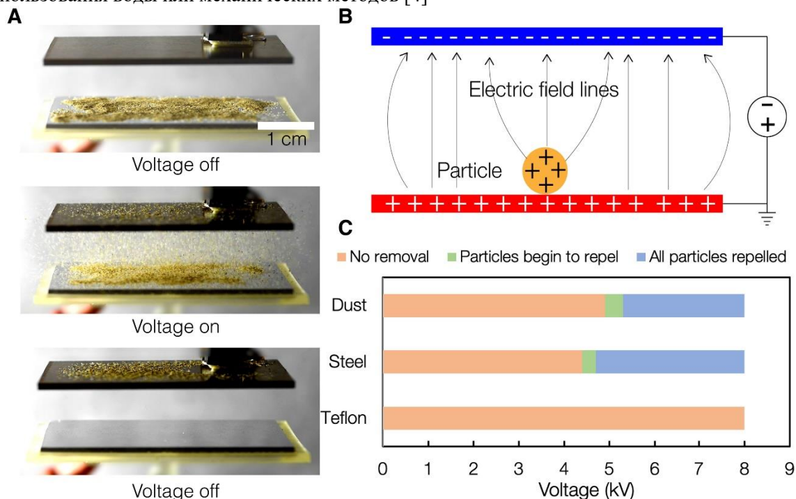
Рис 1. Автоматическое пылеудаление для солнечных панелей с помощью электричества
