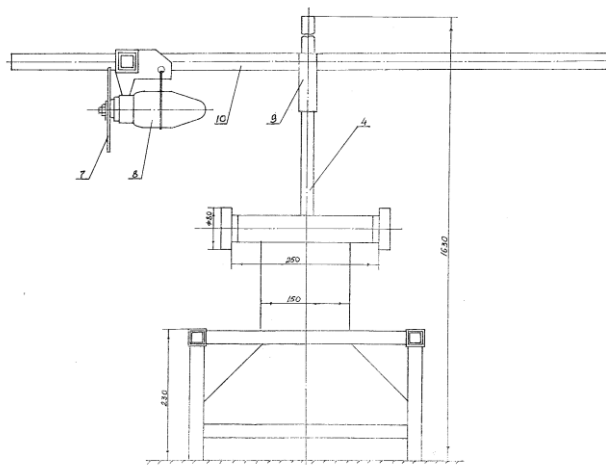
3-сурет. Станоктың бүйірінен көрінісі
