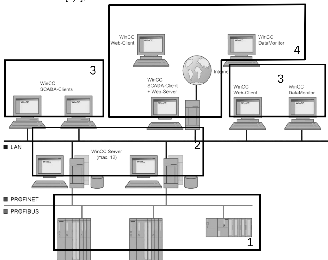
Рисунок 1. Пример принципиальной схемы использования локальной/глобальной сети в производстве
