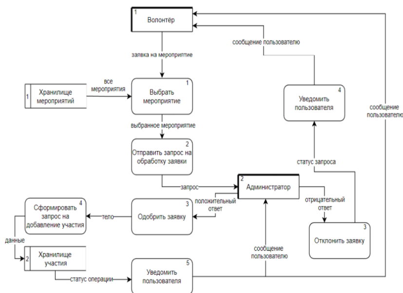
Сурет 2. "Ерікті" пайдаланушының өтінім беру процесінің " DFD "диаграммасы және оны"әкімші" пайдаланушының өңдеуі
