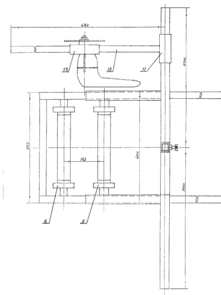
2-сурет. Станоктың төбесінен көрінісі.
