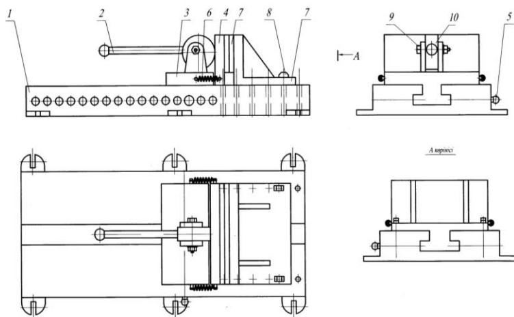
Сурет 1. Металл кескіш станоктарға арналған бөлшектерді бекіткіш сайман.
