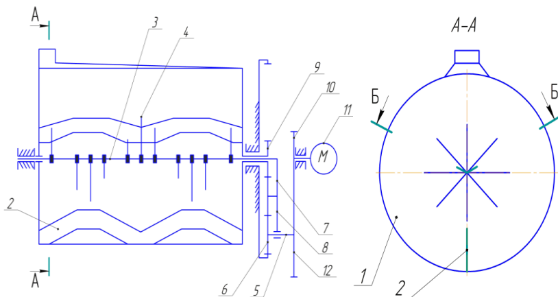
Рисунок 1. Смеситель для приготовления строительных смесей.
