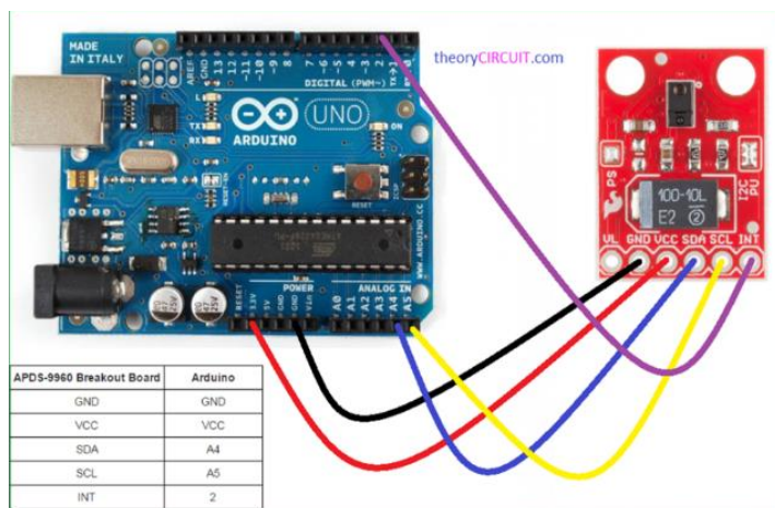
Рисунок 2. Схема подключения на Ардуино.
