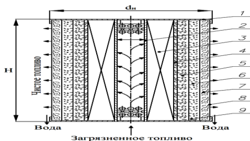
Рисунок 1. Фильтр-водоотделитель.
