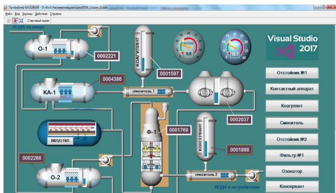
Сурет 1. Trace Mode интегралданған ортасындағы ауызсуды дайындаудың автоматтандырылған басқару жүйесінің схемасы.
