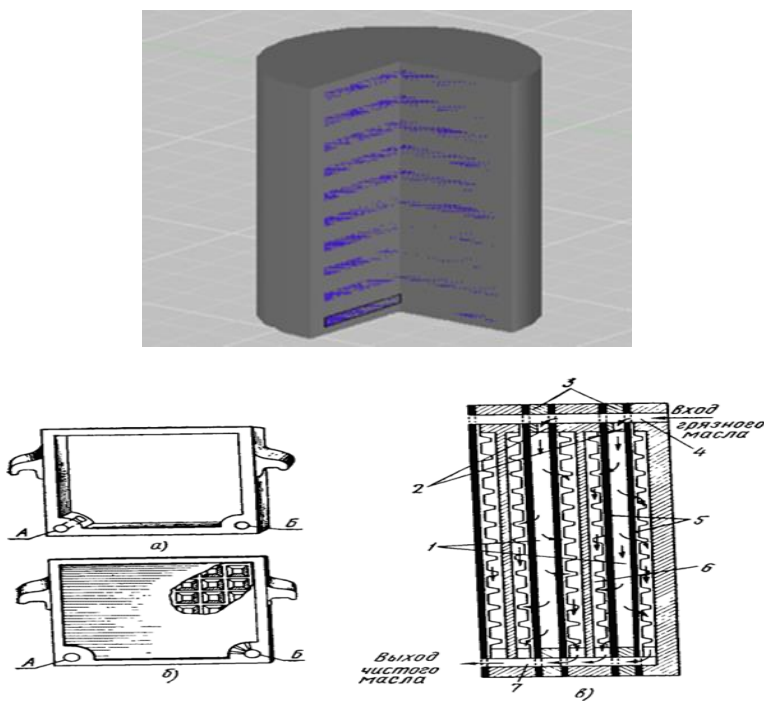
Рисунок 1. Разработанная модель фильтра.
