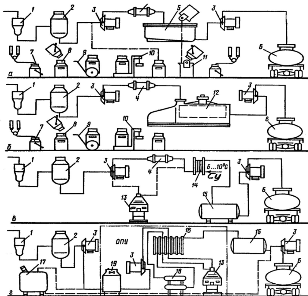
Сурет 1. Сүтті алғашқы өндеу желісінің негізгі технологиялық сұлбалары: а) салқындатылмаған сүтті сүт зауытына өткізу; б) танк-салқындатқышта салқындату; в) пластиналы салқындатқышта сүтті салқындату; г) сүтті пастерлеу
