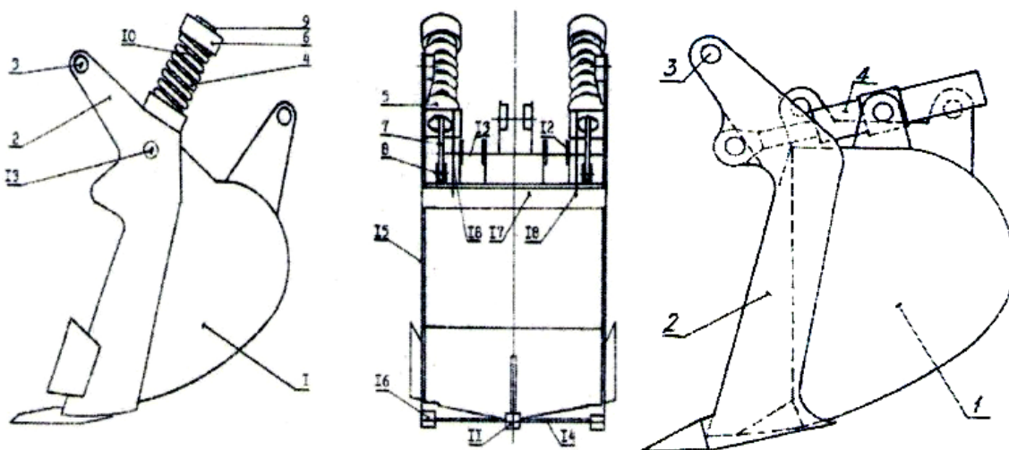
Рисунок 1. Ковш экскаватора с самоприспосабливающейся режущей кромкой
