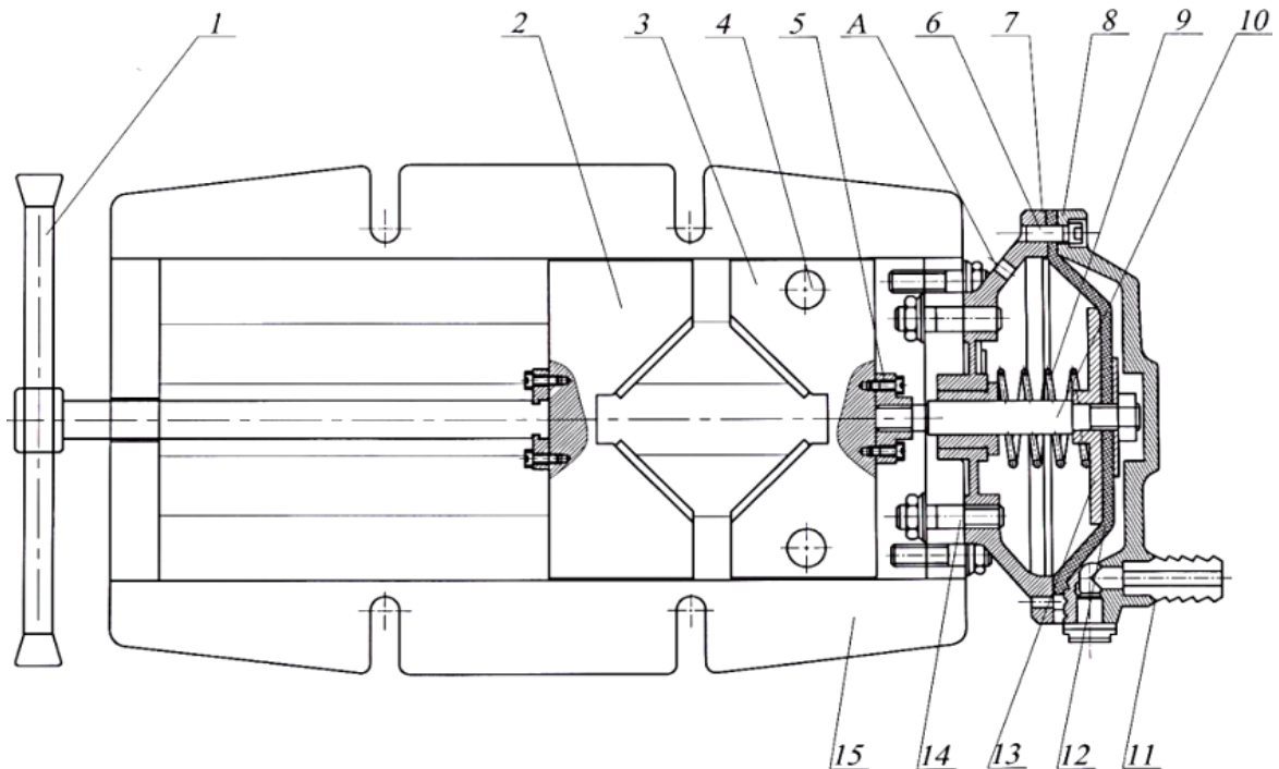
Сурет 1. Цилиндр бетті бөлшектерді центрлеп бекітетін қысқыш сайман
