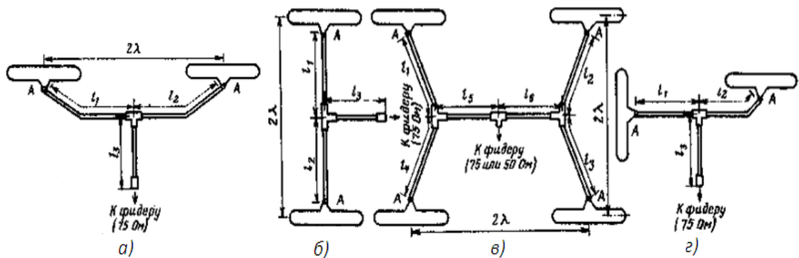
Сурет 1. Антеннаның жүйесін құрастыру
