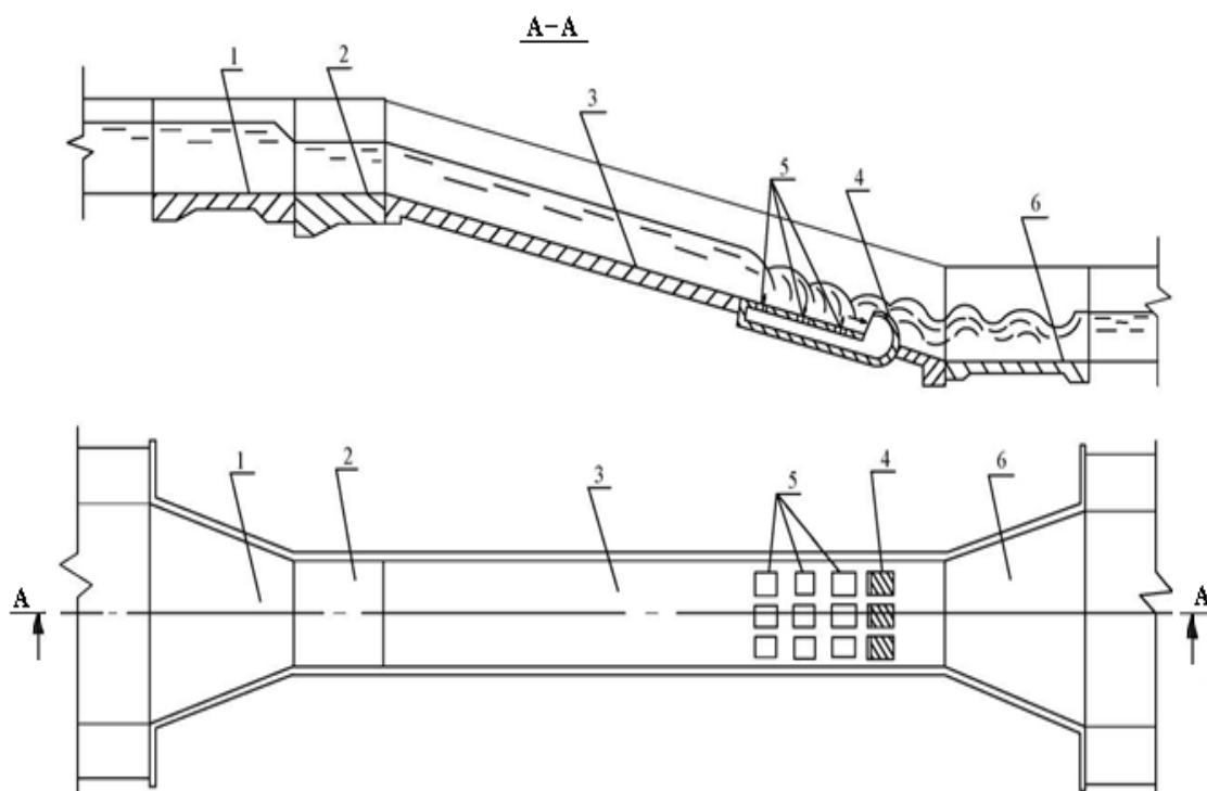
Сурет 1. Құбырлы арын бәсеңдеткішті тезағар
