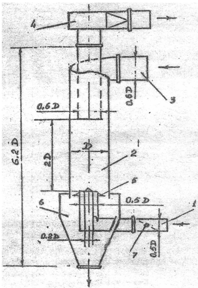
Сурет 1. Гидродинамикалық қарама-қарсы құйынды ВЗП маркалі шағбөлгіші
