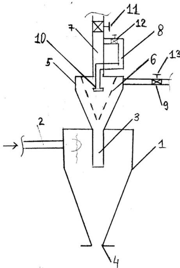
Рис 1. Гидроциклон с камерой дополнительной очистки:
