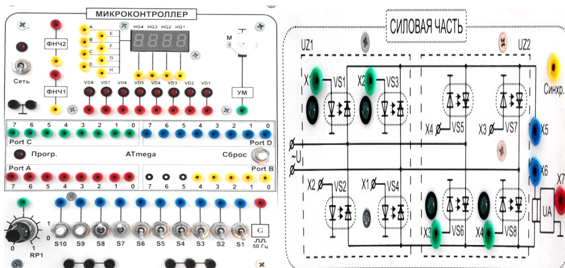
Рис. 1. Модуль микроконтроллерного управления тиристорным преобразователем
