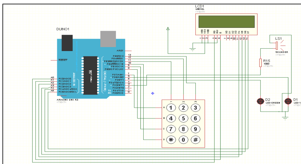
Сурет 1. Дайын кодтық құлып моделінің схемасы
