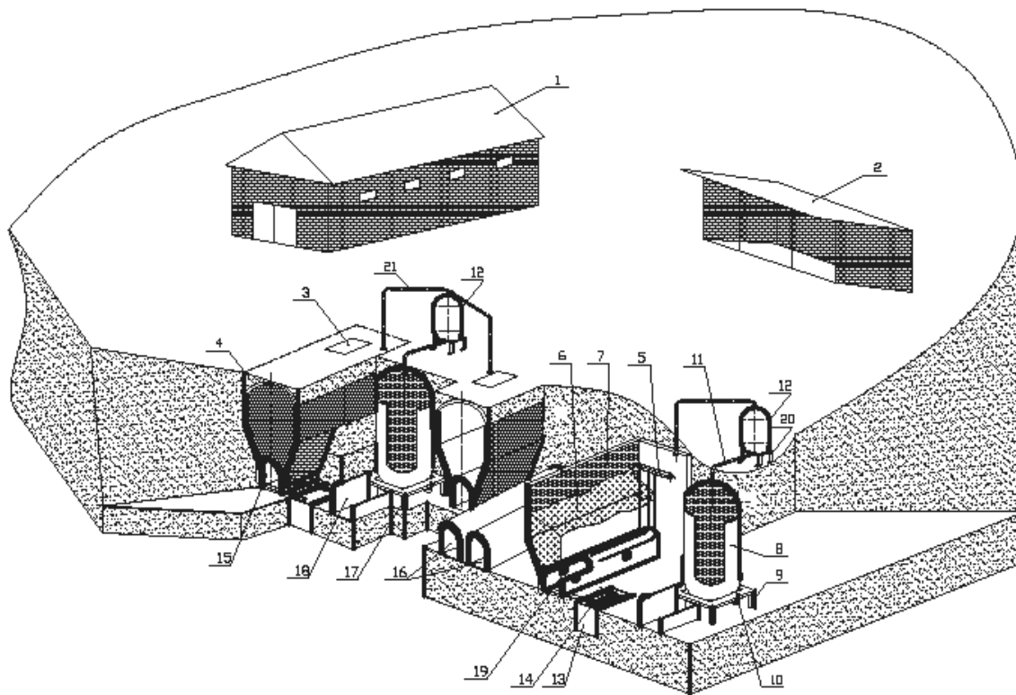
Сурет 1. Жер асты биогаз құрылымы
