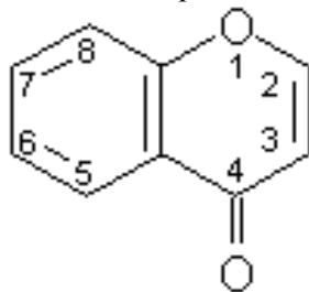
Сурет 1. Бензо-γ-пирон (хромон) туындыларының химиялық құрылысы
