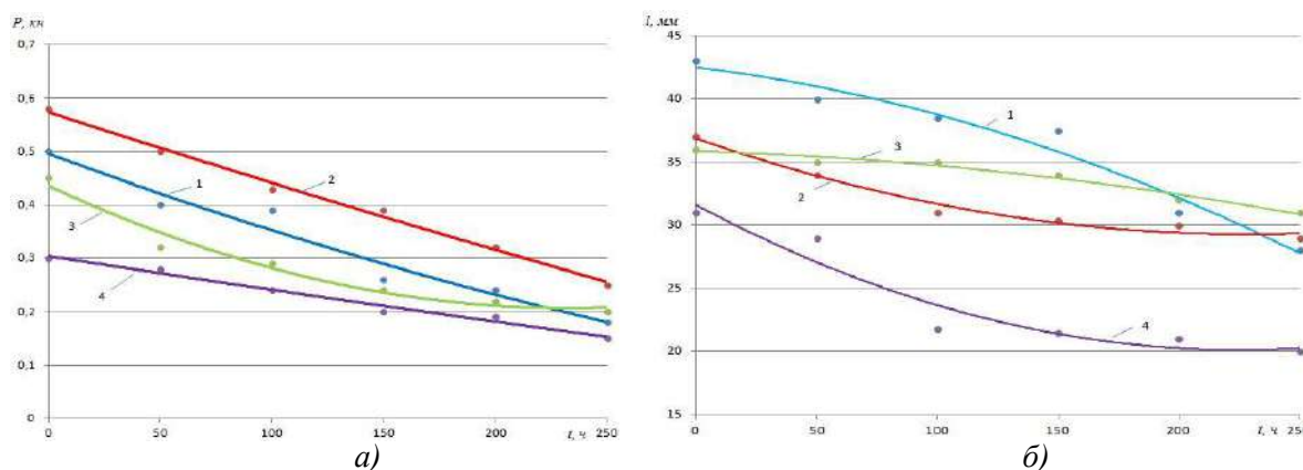
Сурет 1. Судың жіпті тігістің үзілу кезіне әсер ету уақыты (а) және тігістің үзілу кезіндегі ұзаруына әсері (б): 1 – қаймалы бастырма тігіс, 2- қайма тігіс, 3 – бастырма тігіс, 4 – айкаспа тігіс
