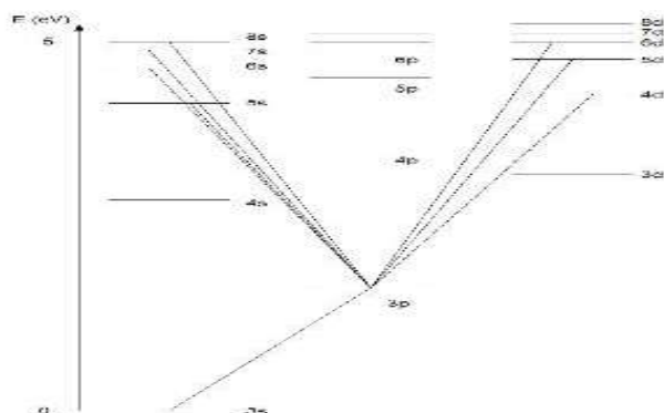
Сурет 2. Натрийдің көрінетін спектрінің готтриандық диаграммасы
